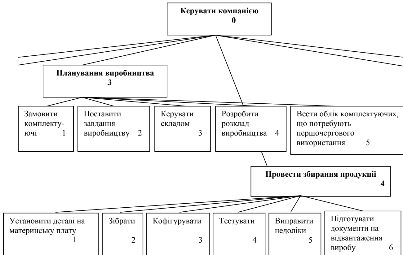
Рисунок 6.2 – Декомпозиція функцій
