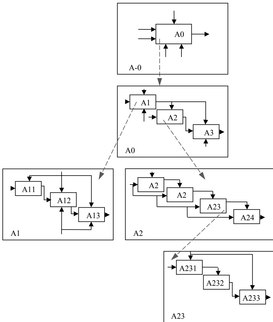
Рисунок 6.3 – Структура IDEF0-моделі
